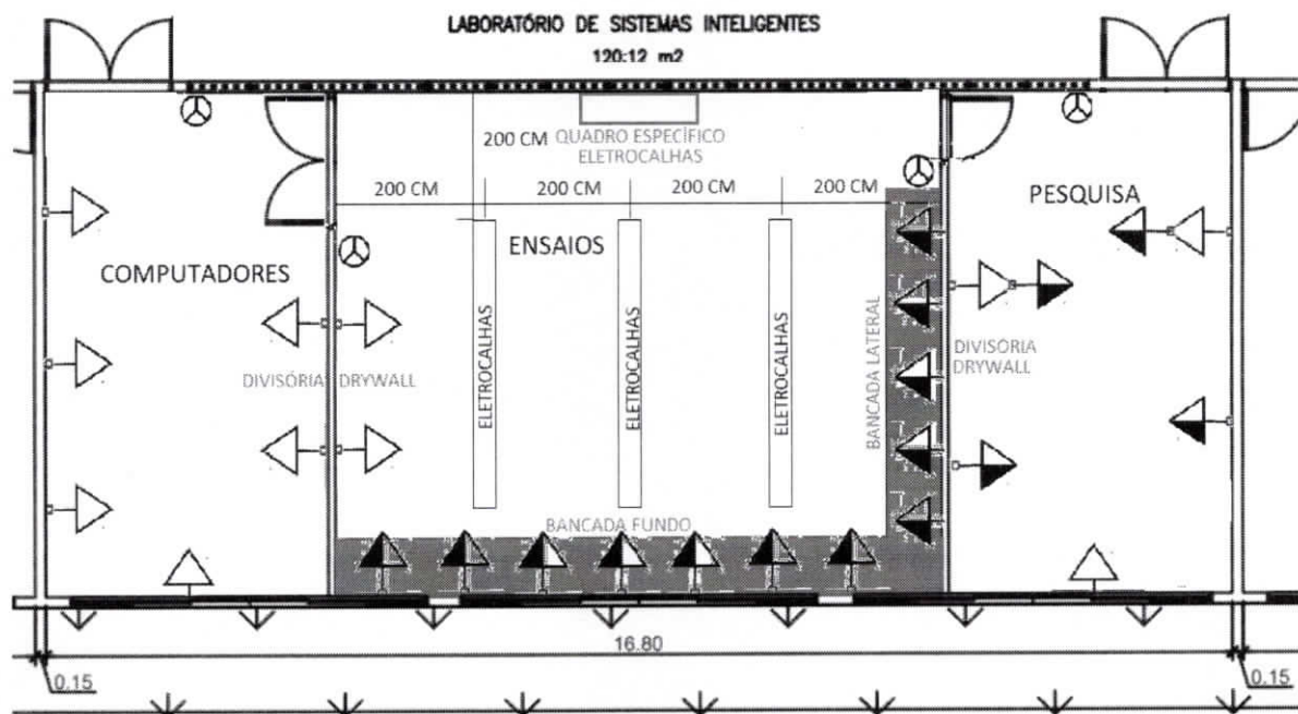
Figura 8 – Planta Baixa do Laboratório de Sistemas Inteligentes.
